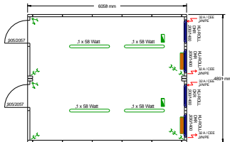
D11 Standardcontainer zur Duoanlage gekoppelt E-Anschluss: 32A/CEE - 3/N/PE E-Heizung: 2 KW
