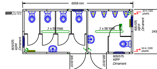
S5 Sanitärcontainer D/H WC E-Anschluss: 32A/CEE - 3/N/PE E-Heizung: 2 KW Frischwasser: 3/4 Zoll Abwasser: DN100
